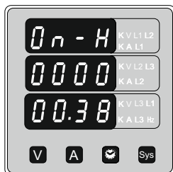
Ekran 8 : Licznik czasu pracy miernika
