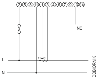
Układ jednofazowy Zasilanie z układu pomiarowego
