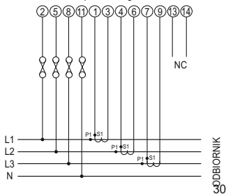
Układ 3-fazowy 4-przewodowy, niesymetryczny Zasilanie z układu pomiarowego
