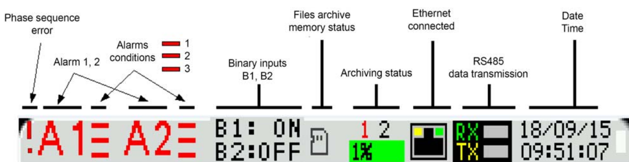
Fig. 10. Information bar
