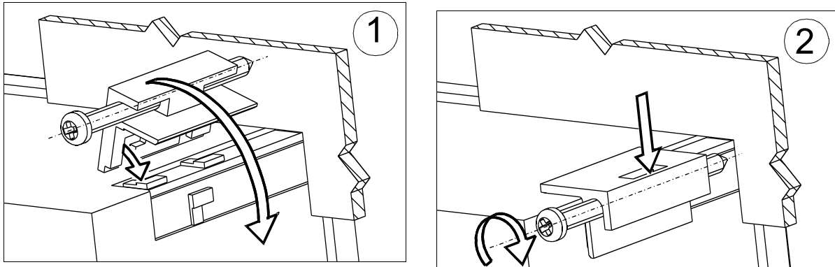
Fig. 2. Meter fitting
