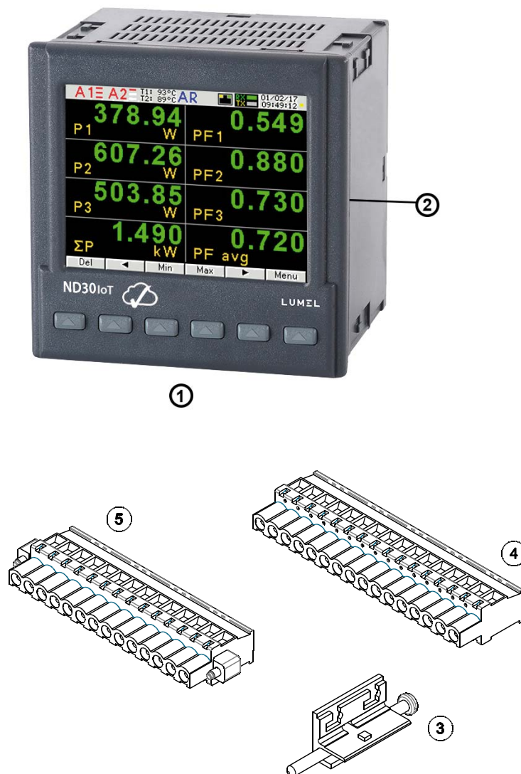
Fig. 1. Meter set
