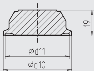
Clamp connection DIN 11864-3
