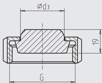
Grooved union nut DIN 11851 with conical coupling, for pipes per DIN 11850
