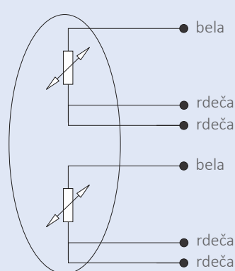
1 x Pt100, Pt1000... 3-vodno
