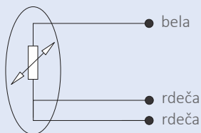
1 x Pt100, Pt1000... 3-vodno
