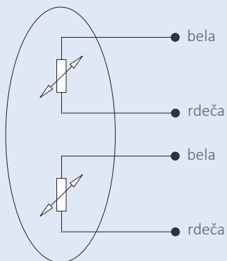
1 x Pt100, Pt1000... 2-vodno
