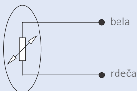
1 x Pt100, Pt1000... 2-vodno
